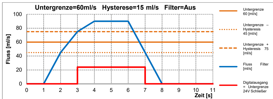
Abbildung 12: Funktion Hysterese beim Grenzwert
