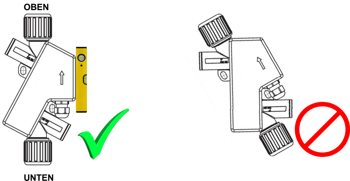
Abbildung 2: Einbaulage des Flowmax 400i
