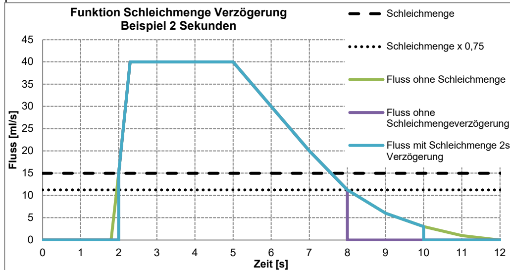
Abbildung 7: Funktion Schleilmengenverzögerung
