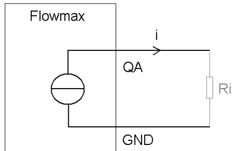
Abbildung 9: Der Stromausgang ist aktiv
